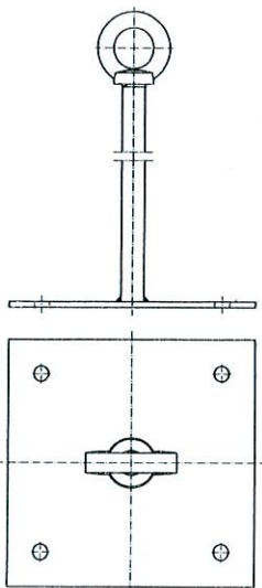
Bild: Anschlagereinrichtung Typ: PREMIUM 4
