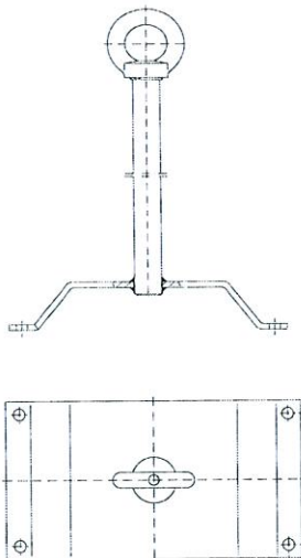
Bild: Anschlagereinrichtung Typ: PREMIUM TRAPEZ
